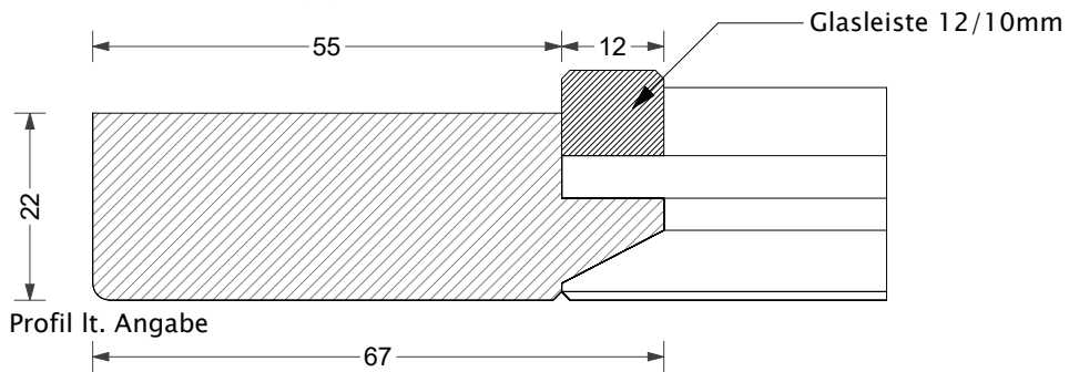
-Ladenfrontfront mit aufrechten Fries (LVB)
