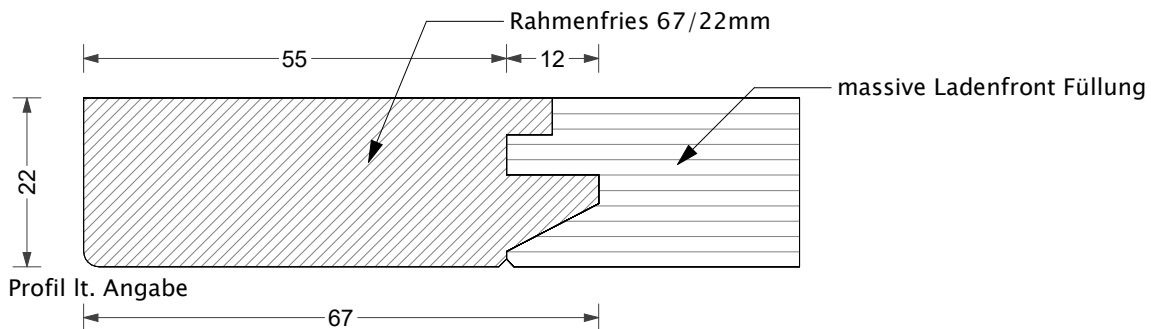
-Ladenfrontfront mit aufrechten Fries (LVB)
