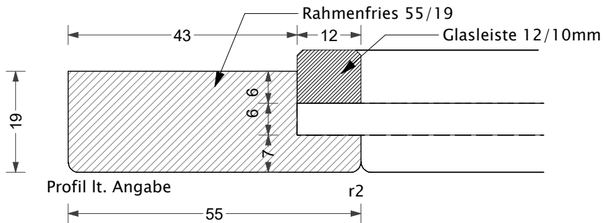
-Glasrahmenfront
