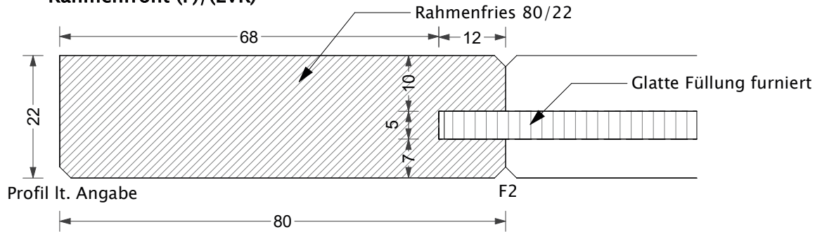
-Rahmenfront (F)/(LVR)
